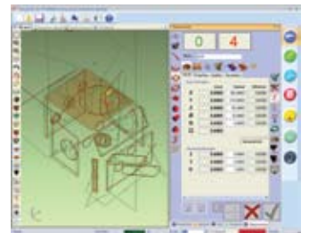
Измерение геометрических объектов с графическим отображением
